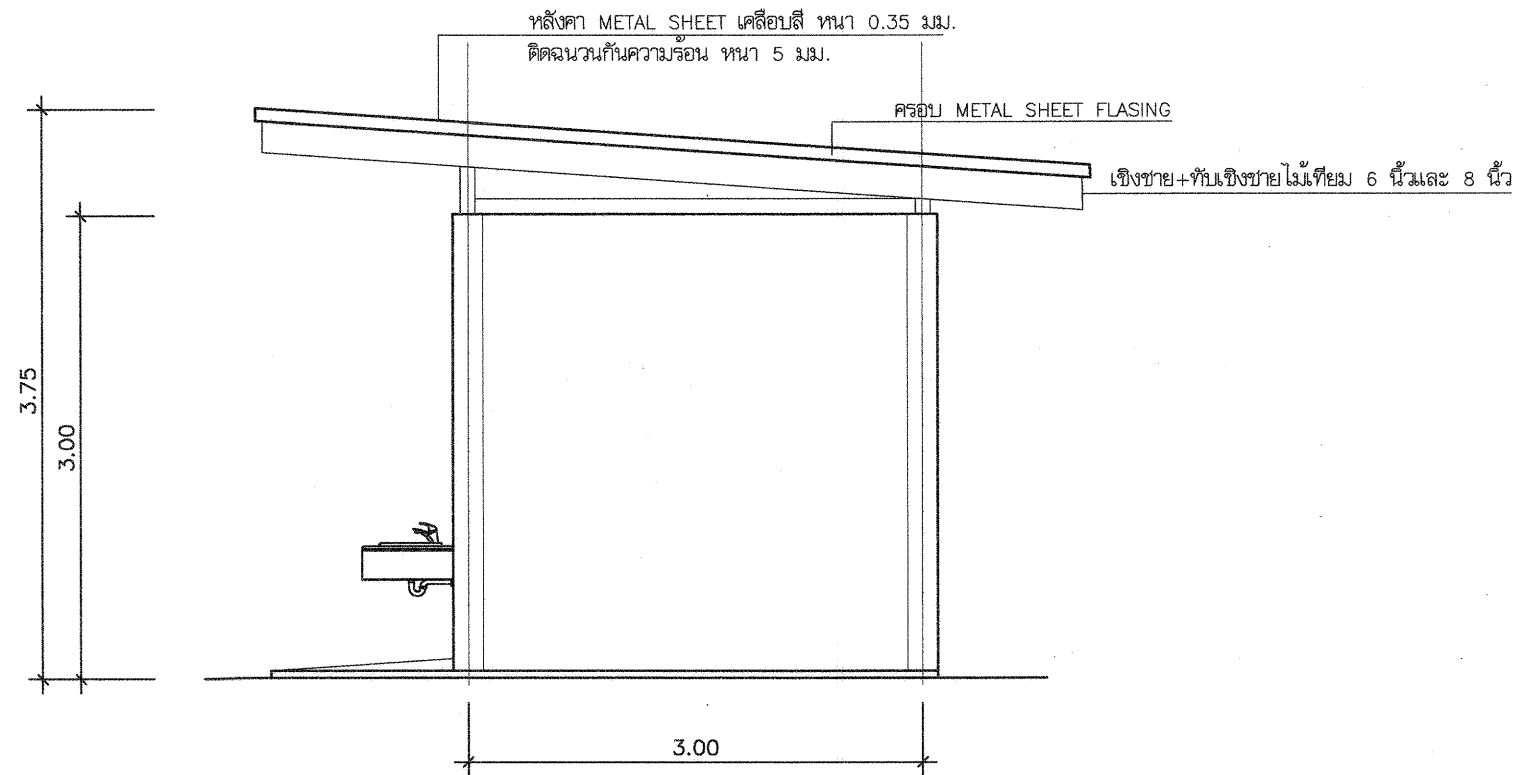
รูปด้านข้าง 4 มาตราส่วน 1:50
