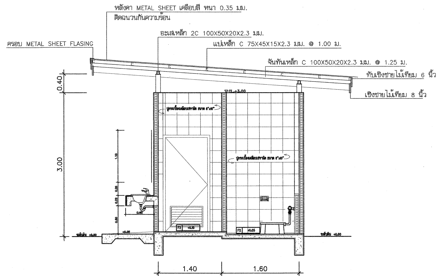
รูปตัด ข-ข มาตราส่วน 1:50
