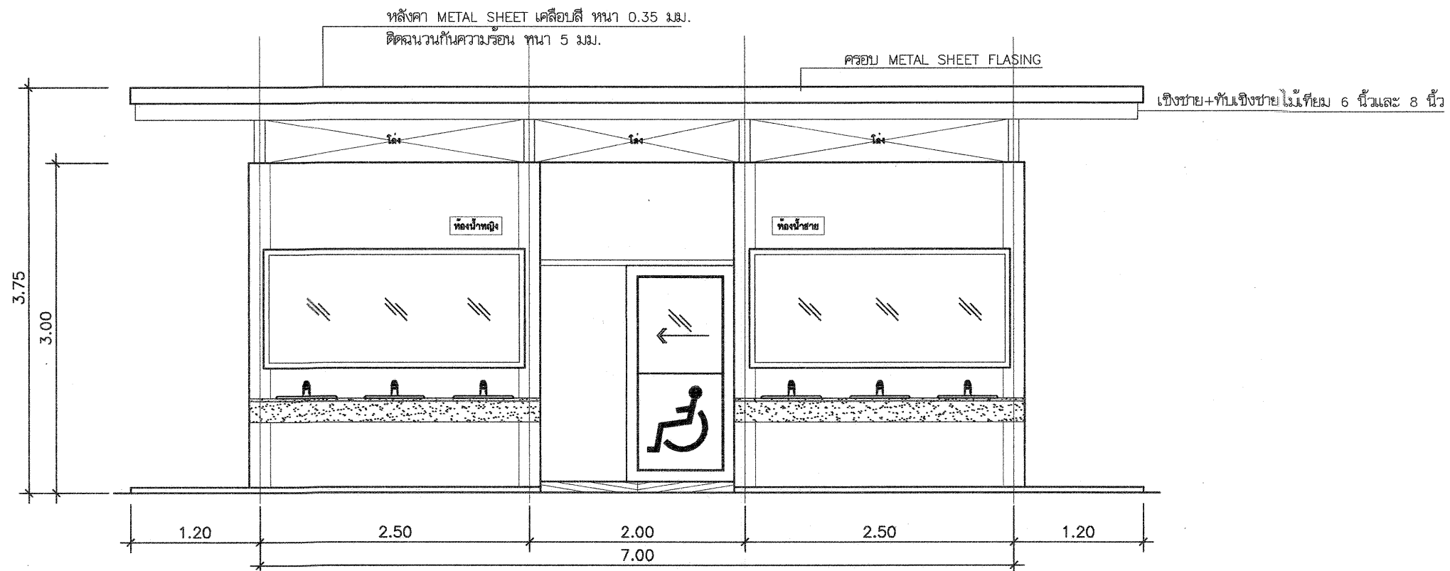
รูปด้านหน้า 1 มาตราส่วน 1:50
